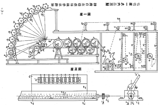
特許第19623号 転換自在捺染緋糸巻機械
