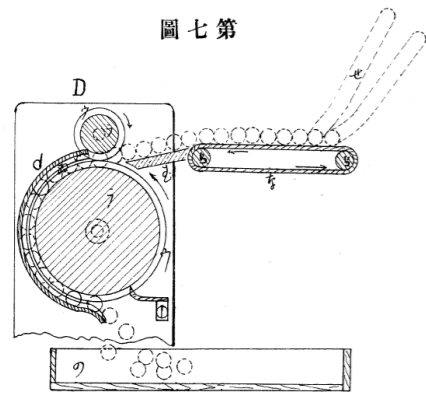
特許第12834号 藤井式製丸機
