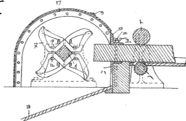
特許第14693号 豆粕粉碎机
